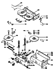
ETB-011616, Normalny mechanizm rozstawiający kompl.
