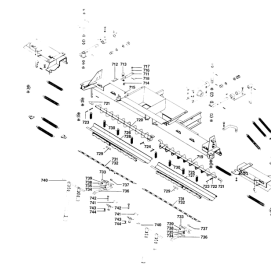
ETB-011623, Ślimak rozstawiający: ślimak, korytko rozstawiające
