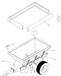
ETB-011603, Rama i zbiornik
