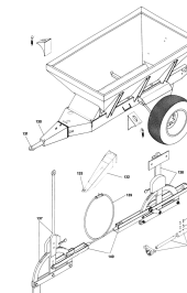
ETB-011607, Dyszle: dyszel pociągowy, ciągnio Bowdena
