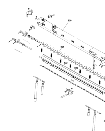
ETB-011626, Ślimak rozstawiający: wysięgnik, korytko rozstawiające
