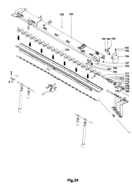
ETB-011624, Ślimak rozstawiający: wysięgnik, łożysko wahiwe
