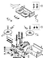
ETB-011617, Normalny mechanizm rozstawiający: wałek wejściowy przekładni
