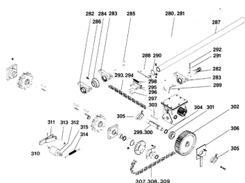
ETB-011612, Wałek napędu głównego i wałek pośredni
