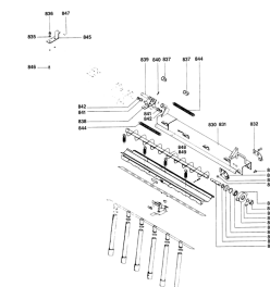
ETB-011627, Ślimak rozstawiający: wysięgnik końcowy
