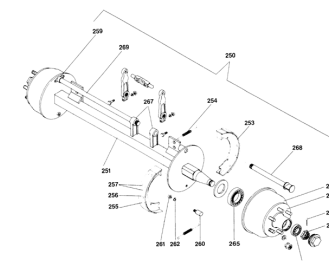
ETB-011611, Oś hamowana (rozstaw kół 1700 mm)
