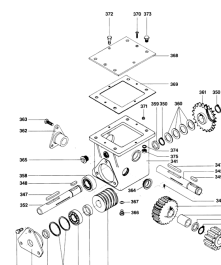
ETB-011614, Przekładnia ślimakowa
