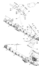
ETB-011621, Ślimak rozstawiający: zawieszenie, osłona przeciwbryzgowa
