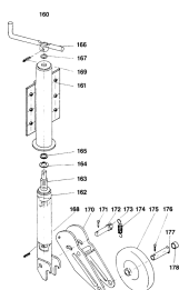
ETB-011608, Podwozie: koło podporowe
