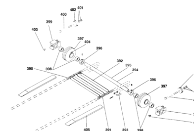
ETB-011615, Ruchoma podłoga i wałek zwrotny
