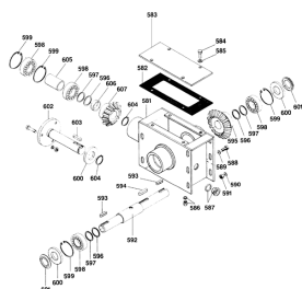
ETB-011620, Wałek wyjściowy przekładni
