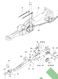
ETB-011606, Dyszle: urządzenie najazdowe, obudowa z kołnierzem
